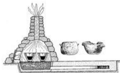
Abb. 2 In einem Schmelzofen wurde über einem Holzkohlefeuer in Tiegeln Metall erhitzt, bis es flüssig war. Um die Temperatur zu erhöhen, wurde durch einen Kanal mit einem Blasebalg Luft in den Ofen gepumpt (die Zeichnung orientiert sich an einer Installation in Tell Qasile aus dem 11. Jh. v. Chr.).
